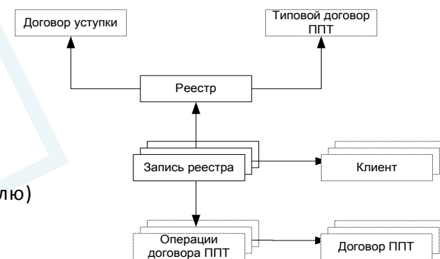
Структура взаимосвязей объектов учета
